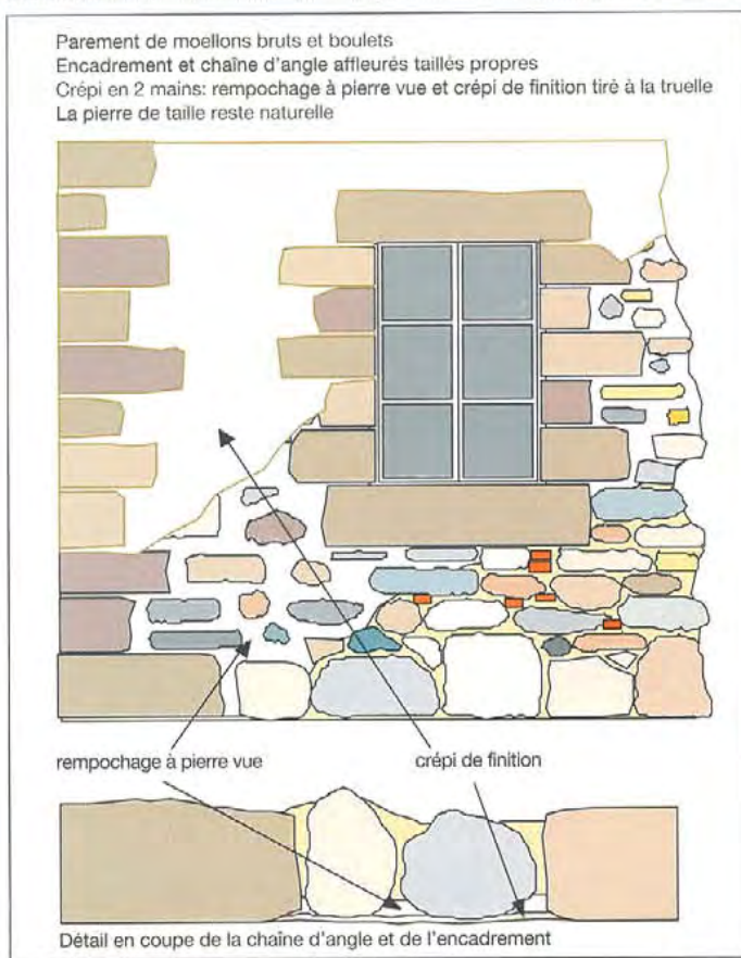
Exemple de composition de crépi
